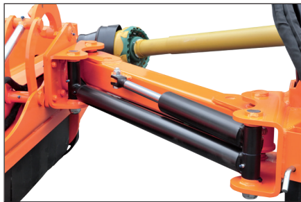
Apsauga nuo kliučių hidraulinio cilindro pagalba
